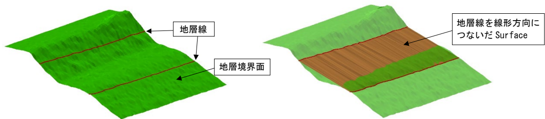
図 4-35 地層線を線形方向につないだサーフェスの例
