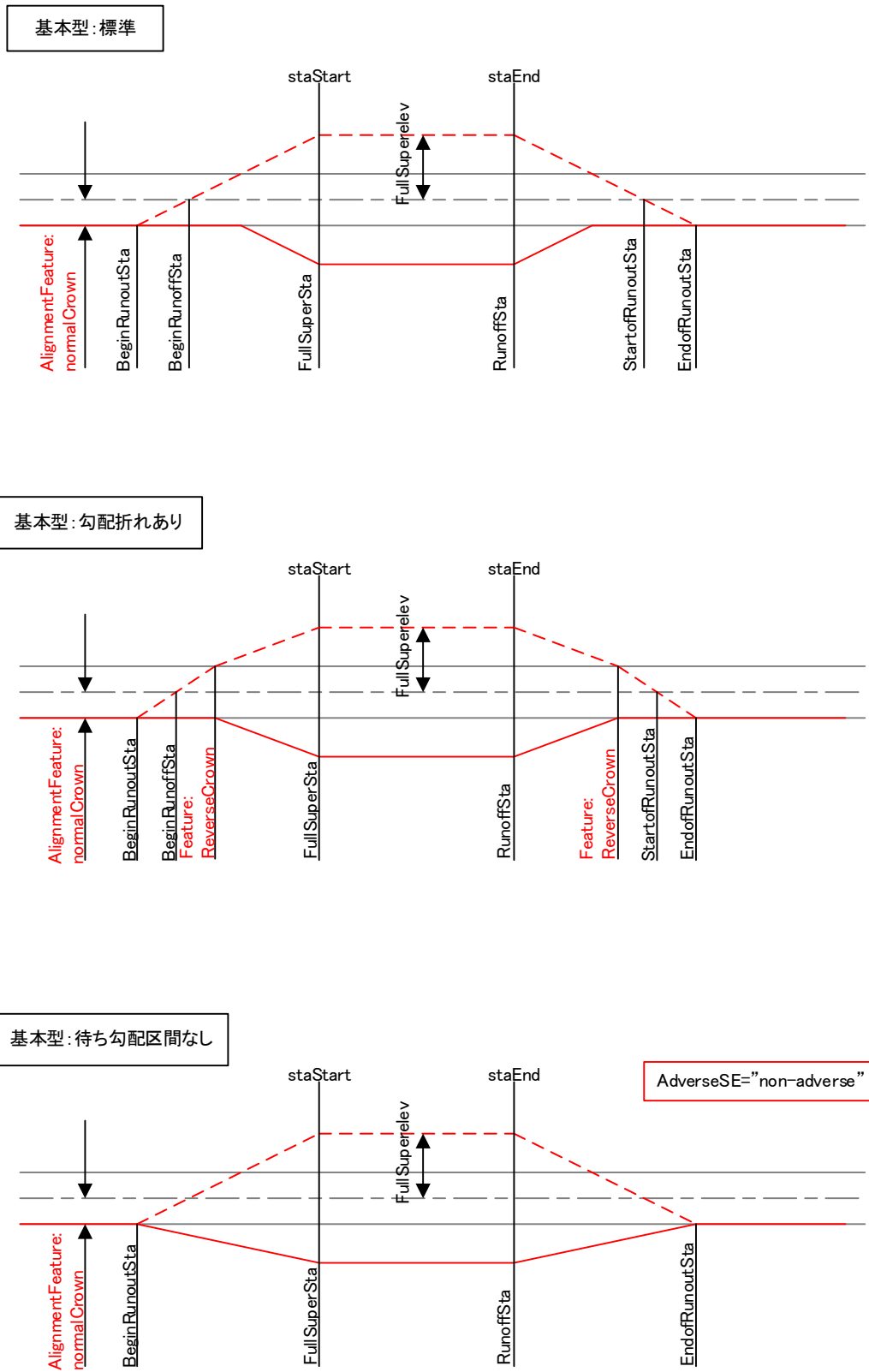
図 4-8 片勾配すりつけの例（基本型）
