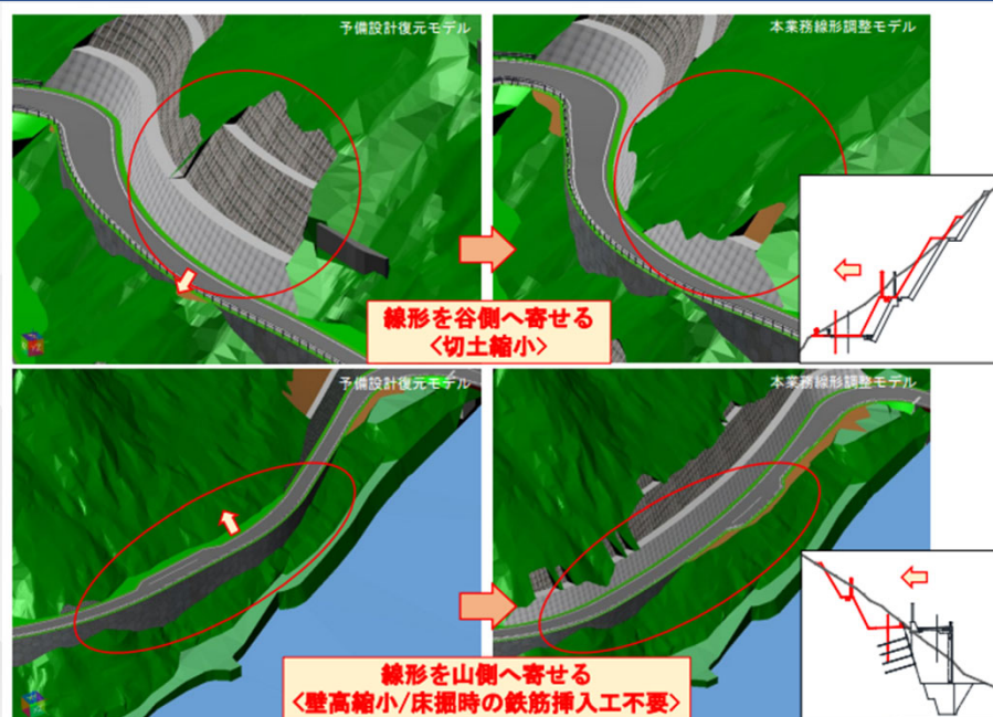
図 3-2 路線選定において活用する BIM/CIM モデルの例
