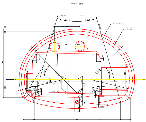
&lt;標準断面図&gt;
