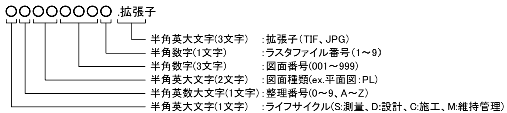
図 2-5 ラスタファイルの命名規則（SXF Ver.3.0 レベル 2 以上の場合）
