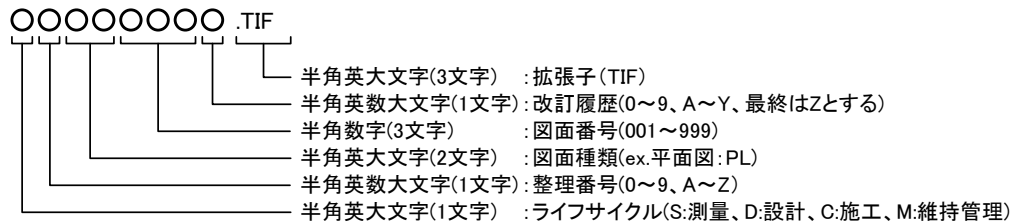
図 2-4 ラスタファイルの命名規則（SXF Ver.2.0 レベル 2 の場合）
